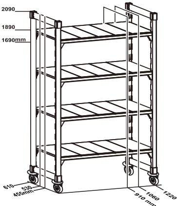
移动式层架
