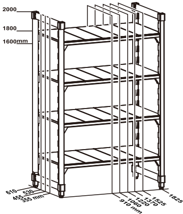
固定式层架
